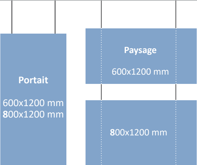
Panneau 2 faces de mousse acoustique 25 mm. A suspendre par câbles traversants. Hauteur réglable. Epaisseur 60 mm.
