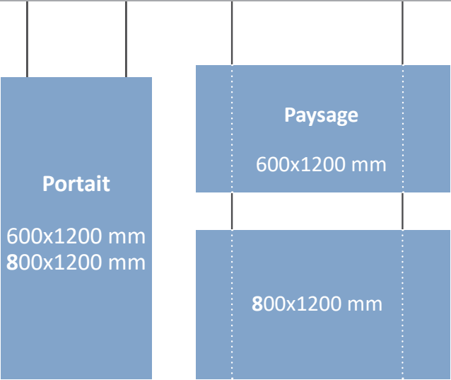
Panneau 2 faces de mousse acoustique 25 mm. A suspendre par câbles traversants. Hauteur réglable. Epaisseur 60 mm.
